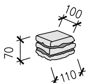
Výplňový blok 11 x 10 x 7 cm
